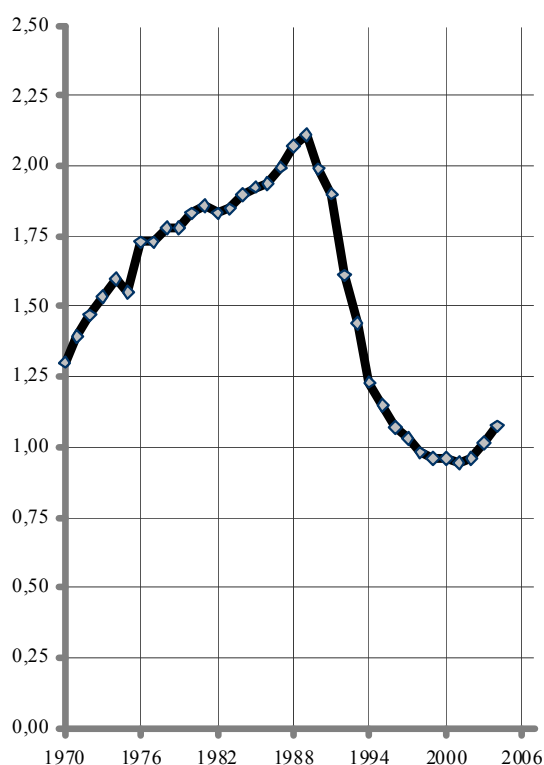
Рис. 3-3. Производительность труда в электроэнергетике РСФСР и РФ (выработка электроэнергии в млн. кВт-час на 1 работника промышленно-производственного персонала).
