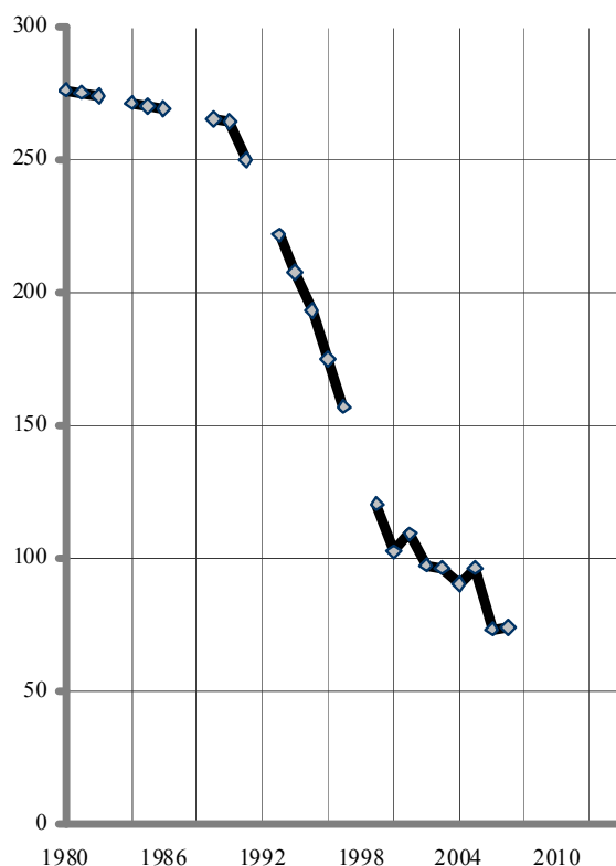
Рис. 3-15. Сокращение производственных мощностей тракторостроения России (тыс. тракторов в год).
